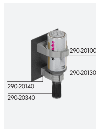
Kettingsmering met ronde borstel en 2 houders
